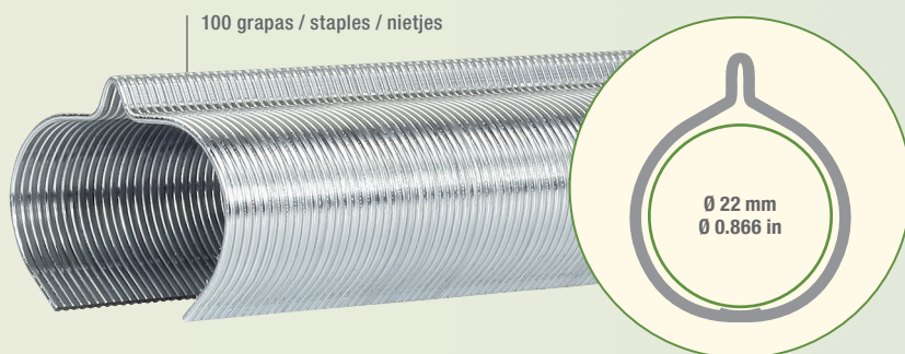
V46 NIETJE Gegalvaniseerd staal
